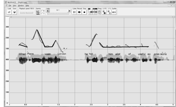
Fig. 5: Prosodic morphing
